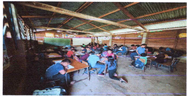
Foto 6: Cambio de vigas de madera por vigas de metal.
